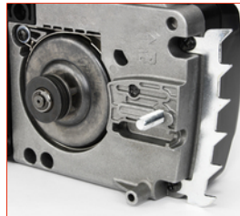
Geschraubte Metall- Zackenleiste für wirkungsvolle Kraftumlenkung und kräfteschonendes Arbeiten
